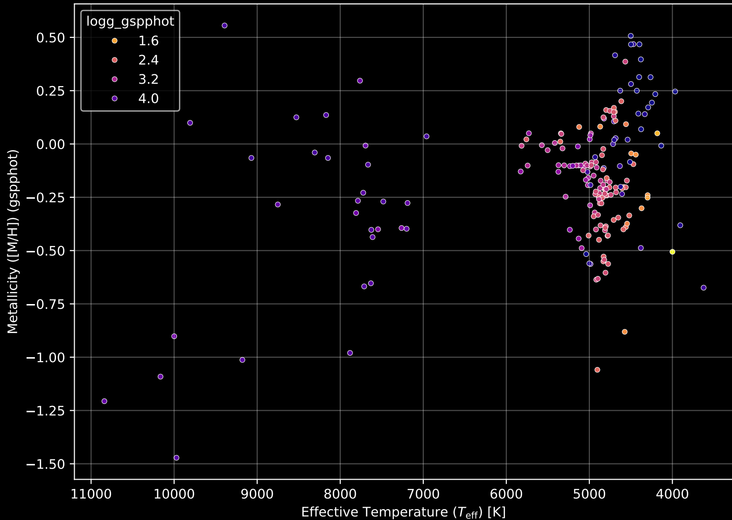
APOGEE DR17 Field: [210+16] Stellar Population Parameters (n= 194)
